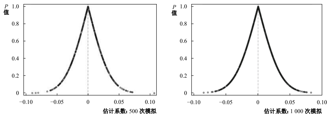
图 3 安慰剂检验
